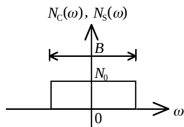
図7 BPF出力雑音のベースバンド電力密度スペクトル
