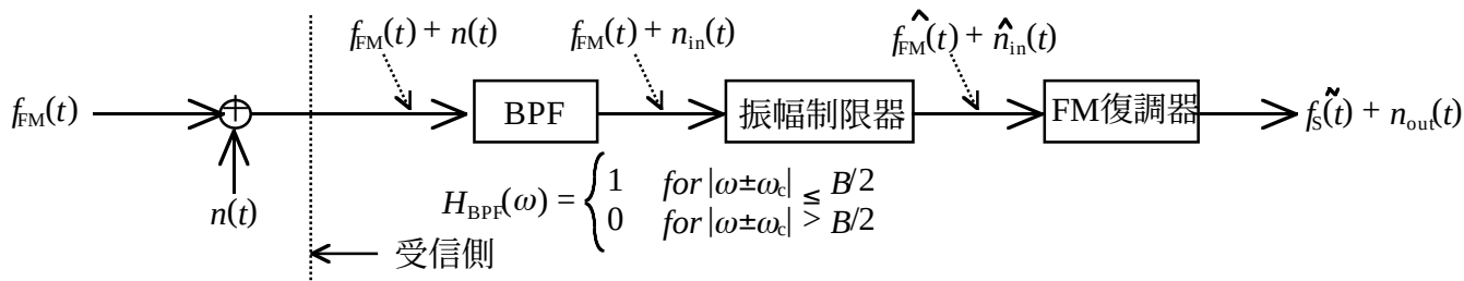
図1 FM信号の復調過程
