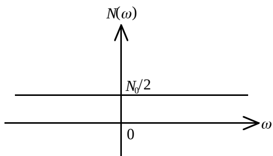
図4 白色雑音 n(t) の電力密度スペクトル
