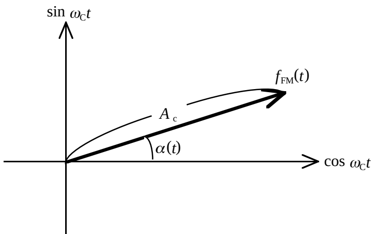
図8 FM信号のベクトル表示
