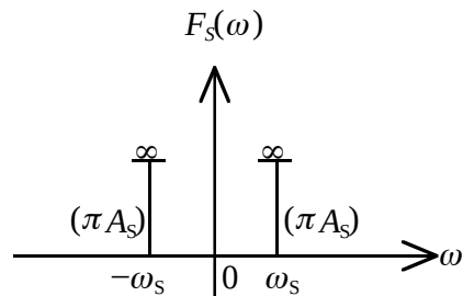
図3 変調信号 f_s(t) の周波数スペクトル密度関数
