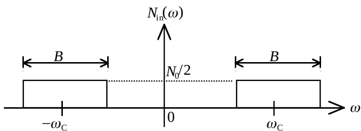
図6 BPF出力雑音 n_{\text{in}}(t) の電力密度スペクトル
