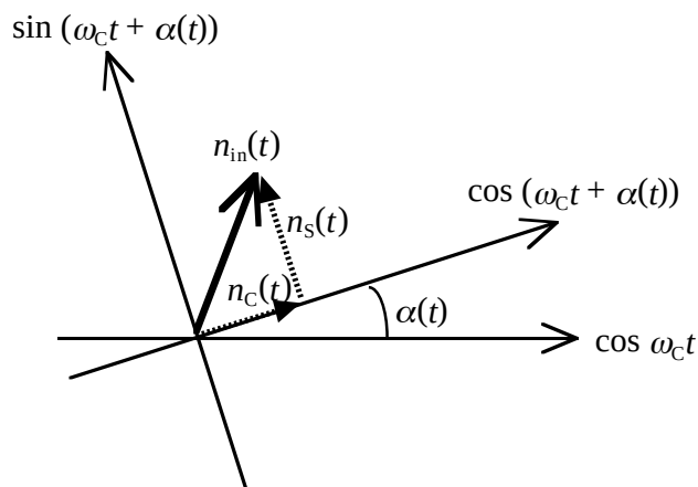
図9 雑音のベクトル表示 (LPF出力)
