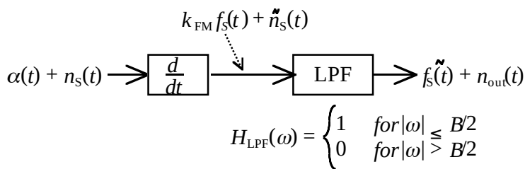
図2 FM復調器
