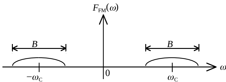
図5 FM信号 f_{\text{FM}}(t) の周波数スペクトル密度関数
